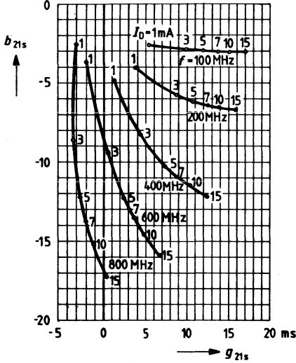
Gate 1 transmittance y_{21s} (source circuit); V_{DS} = 15\text{ V} ; V_{G2S} = 4\text{ V} ; I_{DSS} = 10\text{ mA}
