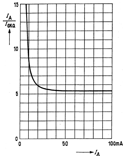
Switching ratio I_A/I_{GKQ} = f(I_A)
