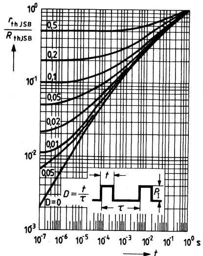
Permissible pulse load \frac{r_{thJSB}}{R_{thJSB}} = f(t) D= parameter
