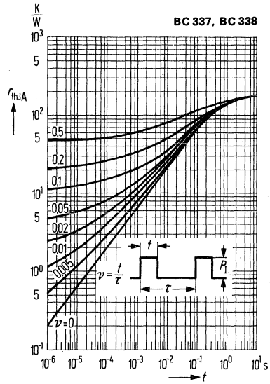
Permissible pulse load r_{thJA} = f(t) v = parameter
