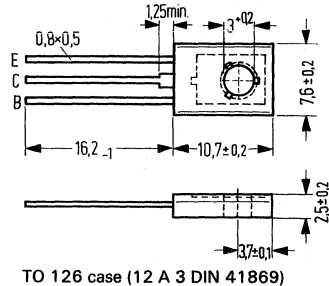
TO 126 case (12 A 3 DIN 41869)
