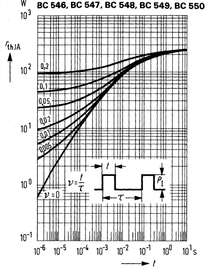
Permissible pulse load r_{thJA} = f(t) v = parameter
