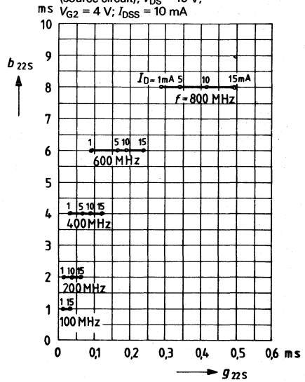
Output conductance y_{22s} (source circuit); V_{DS} = 15\text{ V} ; V_{G2} = 4\text{ V} ; I_{DSS} = 10\text{ mA}
