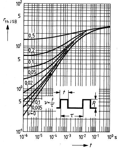
Permissible pulse load r_{thJSB} = f(t) v = parameter
